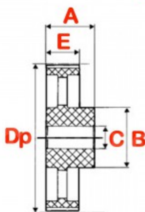
6 F - Type évidé flasqué
