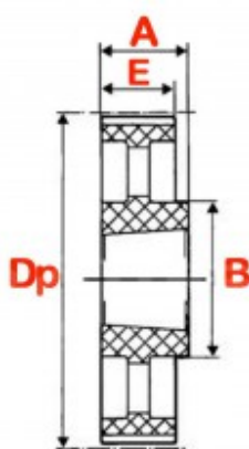
6 M - Type évidé non flasqué en fonte
