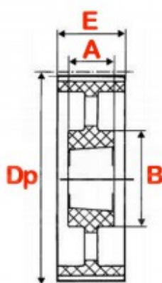
9 M - Type évidé non flasqué en fonte
