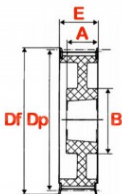
11 M - Type allégé flasqué en acier
