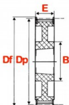
12 MF - Type allégé flasqué en acier
