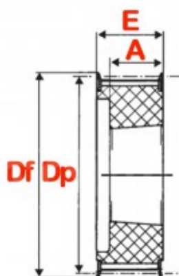
2 MF - Type plein flasqué en acier
