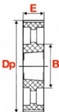
7 M - Type évidé non flasqué en fonte
