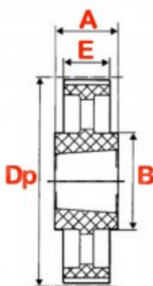
10 M - Type évidé non flasqué en fonte
