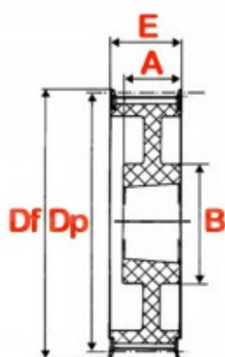
11 MF - Type allégé flasqué en acier
