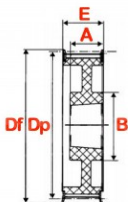
11 MF - Type allégé flasqué en acier
